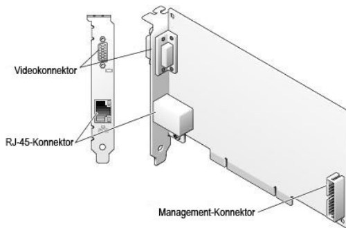
Abbildung 1-2. DRAC 4/I Hardware-Funktionen
